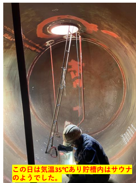
貯槽内に残ったガスを燃焼させる作業 貯槽の開放検査で一番緊張する場面です。
